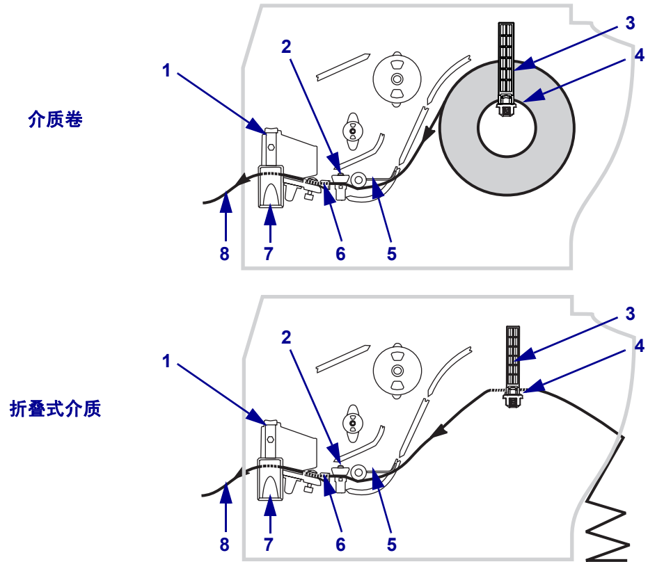
图 17 • 切纸模式
